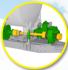
Vakuumpumpe oder Vacu-Storm mit hohem Durchfluss (Durchflussmesser optional)
