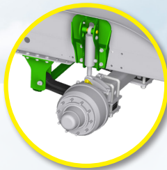
Hydraulische Federung der Deichsel und der Achsen
